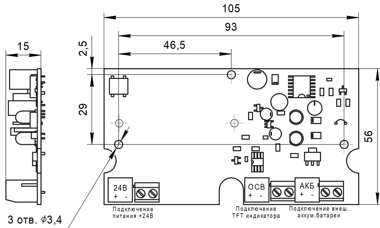
Рис.1 – Внешний вид платы управления аварийным освещением ПУАО НШЕК.468332.007
