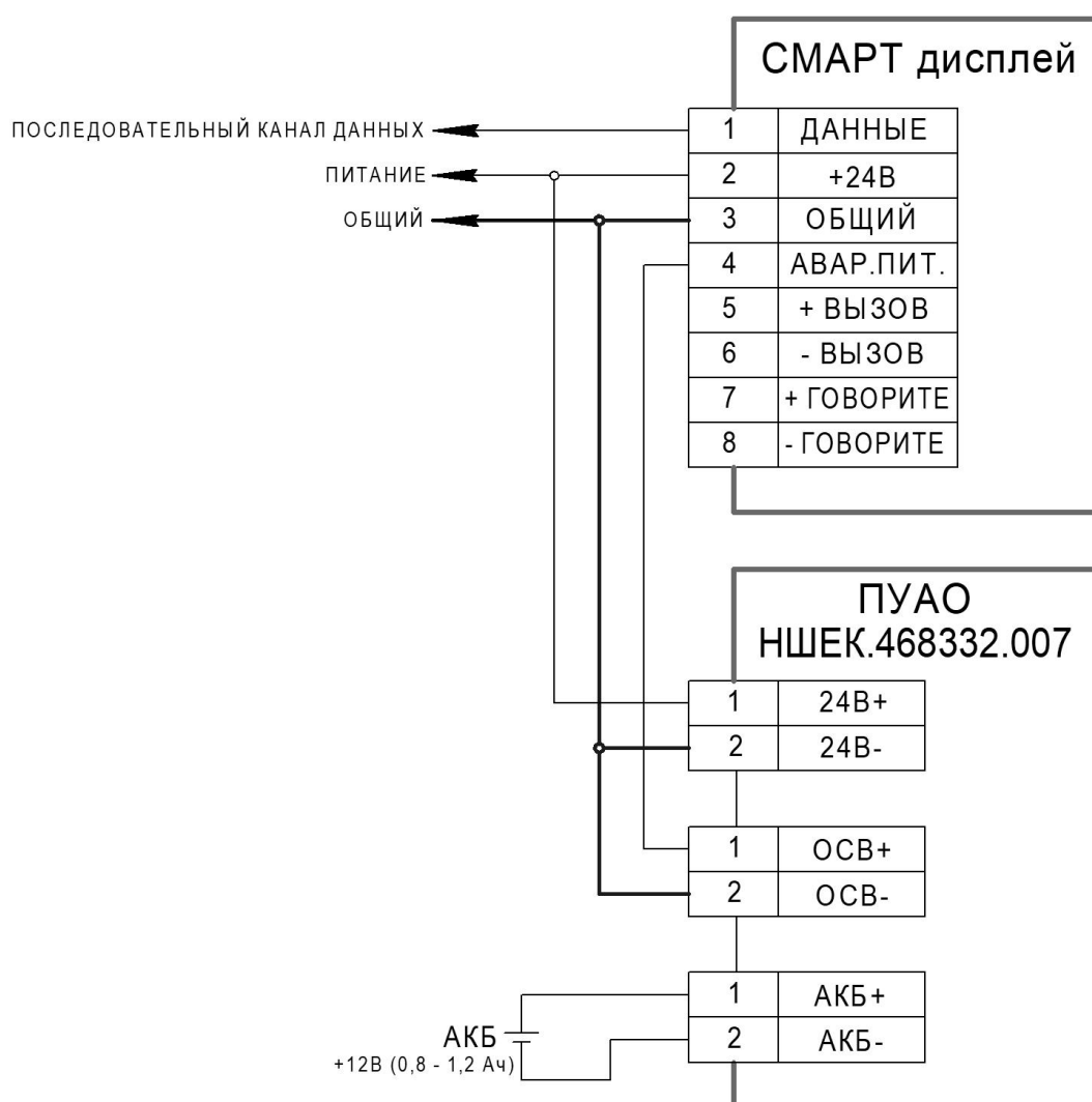
Рис.2 – Схема подключения платы ПУАО НШЕК.468332.007 к дисплею с функцией аварийного освещения
